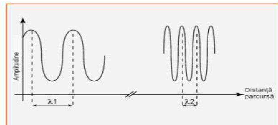
Fig. 1.6. Forma undei de lumină
