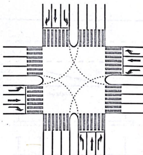
Marcaj de ghidare în intersecție
